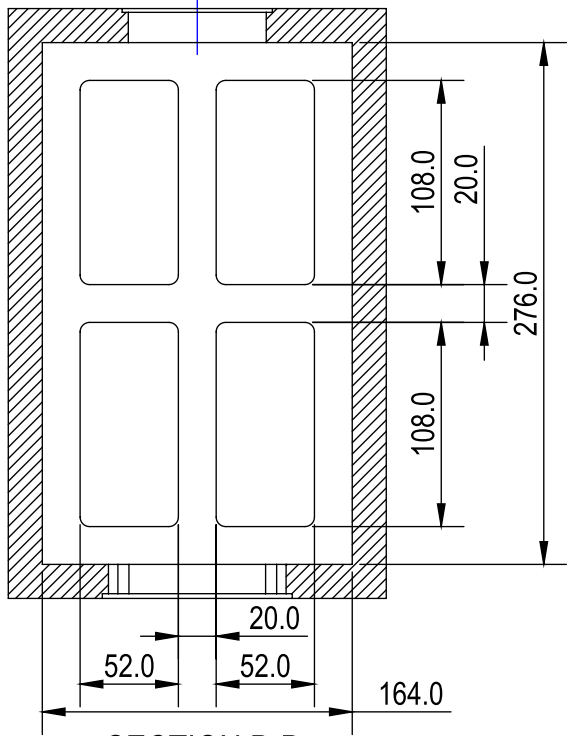
SECTION B-B SCALE 1 : 4
