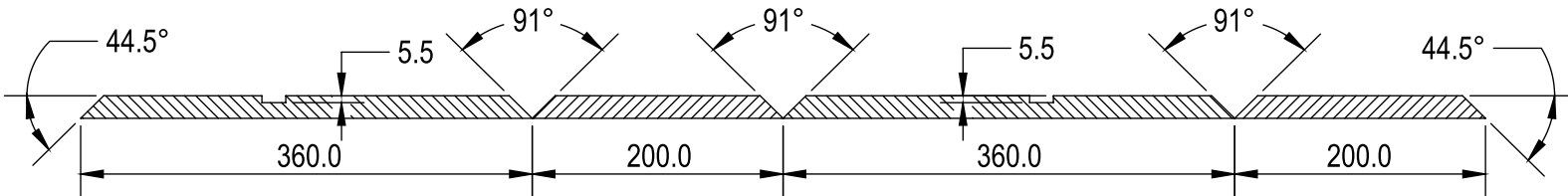
SECTION A-A SCALE 1 : 6
